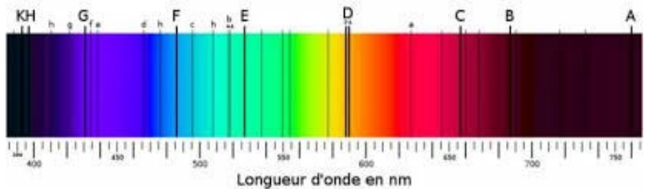
Spectre d'absorption du soleil
