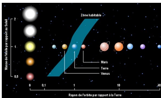
La bande bleue correspond à la zone habitable du système solaire
